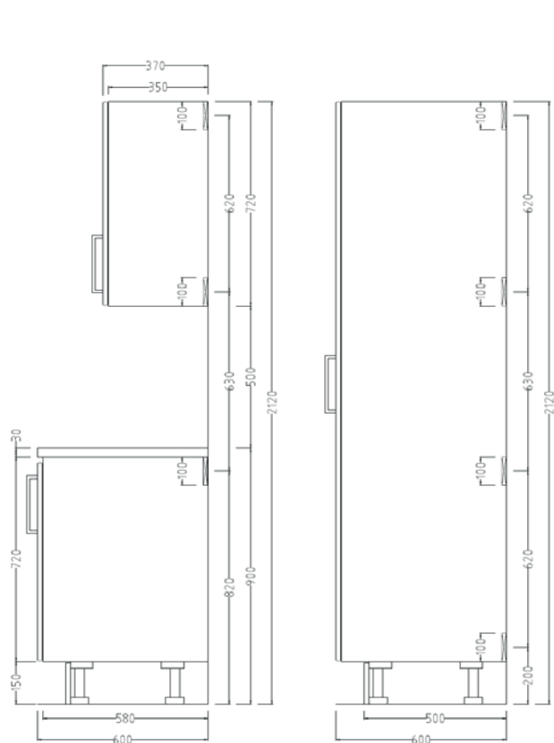
INFÄSTNING INREDNING HÖJD 2100mm
