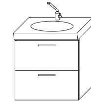
TVÄTTSTÄLLSHURTS VÄGGMONTERAT 2ST LÅDOR L500, 600, 800 H575 D370 1ST TVÄTTSTÄLL (IFÖ SPIRA)
