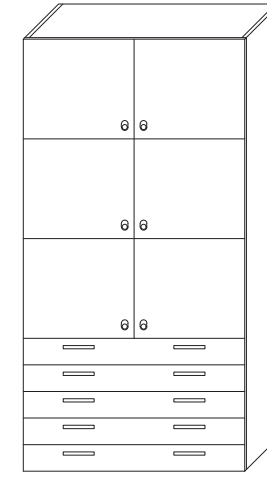
MATERIALSKÅP MS6TSL 6ST TÄCKTA LUCKOR, 5ST LÅDOR L800, 1000 H1950 D450
