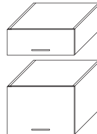
TOPPSKÅP OVAN KYL/FRYS 1ST ÖVERKANT'S HÄNGD LUCKA L600 H230, 430 D600
