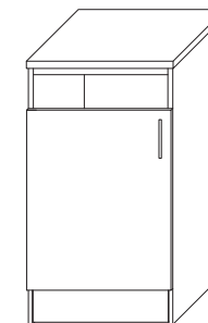
AVFALLSKÅP MED SÄCKHÅLLARE ÖPPNING FRAM ALT I TOPPSKIVA L600 H870, 1070 D600
