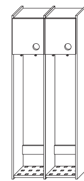
KAPPRUMSSKÅP VÄGGHÄNGD ALT. GOLVSTÄNDE MED ELLER UTAN SITTBÄNK, LUCKA MED 60mm HÅL 2ST ANKARKROKAR SKOHYLLA I ROSTFRI PLÅT L300, 600, 900, 1200 H1500, 1650 D250
