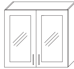
VÄGGSKÅP GLASADE PARLUCKOR L600, 800, 1000 H700, 900 D370
