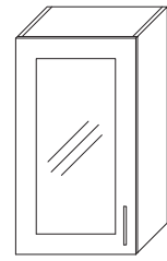
VÄGGSKÅP 1ST LUCKA L300, 400, 500, 600 H700, 900 D370
