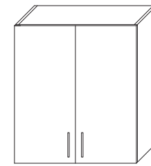
VÄGGSKÅP PARLUCKOR L600, 800, 1000 H700, 900 D370
