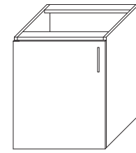
BÄNKSKÅP/DISKBÄNKSSKÅP 1ST LUCKA L300, 400, 500, 600 H520, 720 D600
