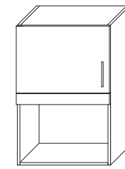
VÄGGSKÅP FÖR MICRO 1ST LUCKA (ÄVEN TOPPHÄNGD LUCKA) L500, 600 H700, 900 D370
