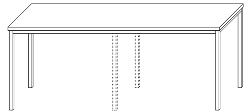
ARBETSBORD TOPPSKIVA MED HÖGTRYCKSLAMINAT BENSTATIV ROSTFRITT ELLER LACKERAT L1000-3000 B500-1240 H350-1100 (ALLA BORD ÖVER L2000 BEHÖVER STÖDBEN PÅ MITTEN)
