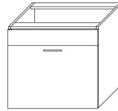
DISKBÄNKSURTS L600, 800 H520, 720 D600 UTDRAG MED SOPKÄRL FAST ÖVRE FRONT
