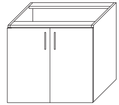
BÄNKSKÅP/DISKBÄNKSSKÅP PARLUCKOR L600, 800, 1000 H520, 720 D600
