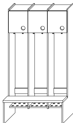
KAPPRUMSSKÅP VÄGGHÄNGD ALT. GOLVSTÅENDE MED ELLER UTAN SITTBÄNK, LUCKA MED 60mm HÅL 2ST ANKARKROKAR SKOHYLLA I ROSTFRI PLÅT L300, 600, 900, 1200 H1500, 1650 D250
