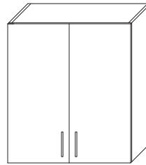
VÄGGSKÅP PARLUCKOR L600, 800, 1000 H700, 900 D370
