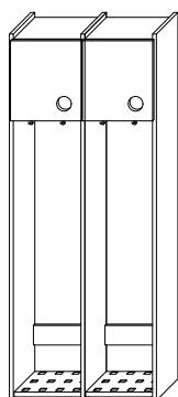
KAPPRUMSSKÅP VÄGGHÄNGD ALT. GOLVSTÅENDE MED ELLER UTAN SITTBÄNK, LUCKA MED 60mm HÅL 2ST ANKARKROKAR SKOHYLLA I ROSTFRI PLÅT L300, 600, 900, 1200 H1500, 1650 D250
