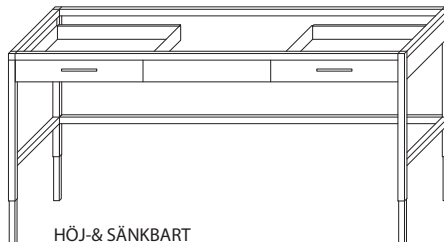
HÖJ- & SÄNKBART ROSTFRITT STATIV HYDRAULSTYRT GÅR ATT VÄLJA MED OCH UTAN LÅDOR MÅTT EFTER ÖNSKEMÅL BÄNKYTA LAMINAT ELLER ROSTFRITT
