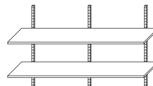
VÄGGHYLLOR I LAMINAT MONTERAT PÅ VÄGGSKENA & KONSOL L400-3000 B150-500 H200-2500(VÄGGSKENA)
