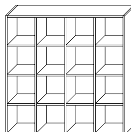
SKOHYLLA/BOXFÖRVARING MODUL HÖJD 2X2 FACK, H550 B550 D270 MODUL HÖJD 2X4 FACK, H550 B1080 D270 MODUL HÖJD 4X4 FACK, H1080 B1080 D270 FACK H250 B250 D250 TILLVAL: PLYWOODLÅDA MED LAMINAT H240 B240 D240
