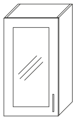
VÄGGSKÅP 1ST LUCKA L300-500 H700,900 D370
