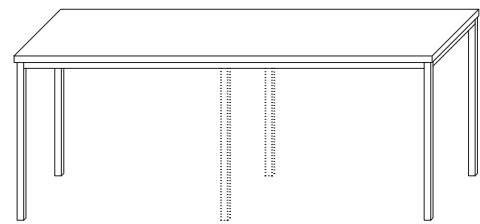
ARBETSBORD TOPPSKIVA MED HÖGTRYCKSLAMINAT BENSTATIV ROSTFRITT ELLER LACKERAT L1000-3000 B500-1250 H350-1100 (ALLA BORD ÖVER L2000 BEHÖVER STÖDBEN)
