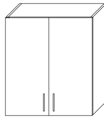
VÄGGSKÅP PARLUCKOR L800-1000 H700,900 D370
