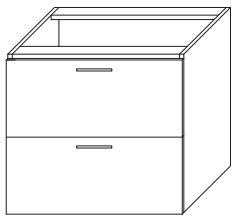
LÅDHURTS/GRYTSKÅP L300-800 H720 D600
