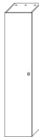
ELEVSKÅP, VENTILERAT MED HÅL I TAK/BOTTENSKIVA 1ST/2ST LUCKA MED HÄNGLÅSVRED 1ST/2ST HYLLA 2ST/4ST ANKARKROKAR L300-400 H1800 D400
