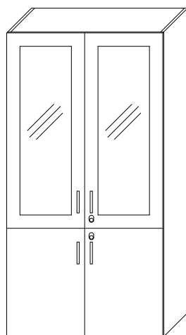
MATERIALSKÅP MS4TG 2ST TÄCKTA 2ST GLASADE LUCKOR L800-1000 H1950 D450
