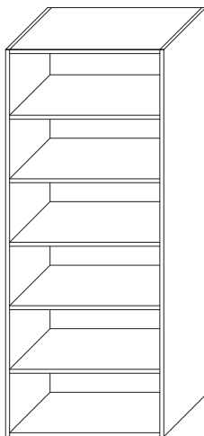
HÖGSKÅP ÖPPET L400,600,800,1000 H1950,2150 D600MM
