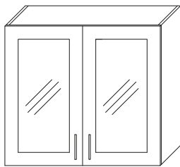
VÄGGSKÅP GLASADE PARLUCKOR L800-1000 H700,900 D370
