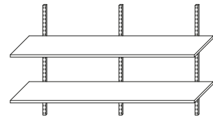
VÄGGHYLLOR I LAMINAT MONTERAT PÅ VÄGGSKENA & KONSOL L400-3000 B150-500 H200-2500(VÄGGSKENA)
