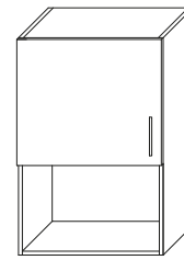
VÄGGSKÅP FÖR MICRO 1ST LUCKA (ÄVEN TOPPHÄNGD LUCKA) L500-600 H700,900 D370
